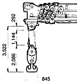
200 t フック
