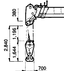
80 t フック
