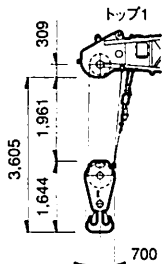
80 t フック
